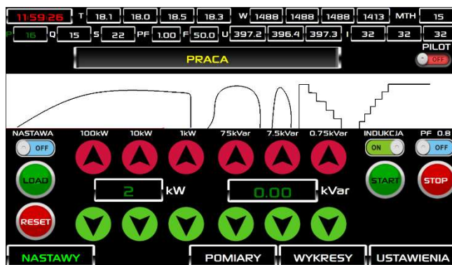
EKRAN POMIARÓW
